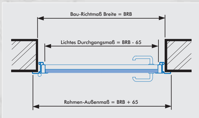
Horizontalschnitt AL-Tür Typ ISO 20 – Außenanschlag
