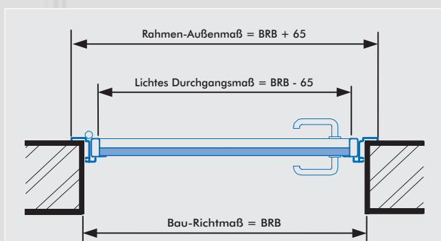
Horizontalschnitt AL-Tür Typ ISO 20 – Innenanschlag
